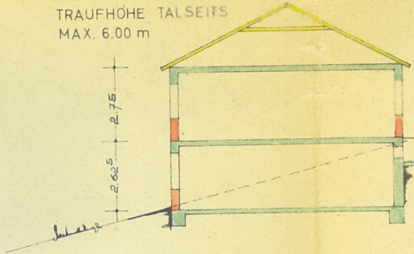
1 1/2 GESCHOSSIG E+U
